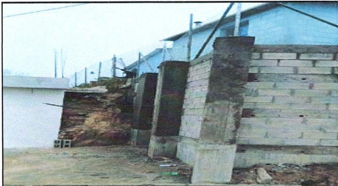
Foto 1: Se aprecia la finalización del mejoramiento de muro de contención suroeste.
