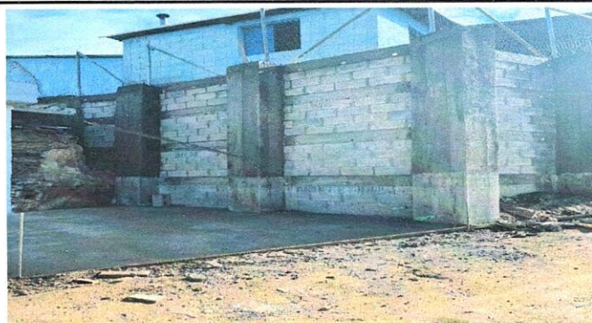
Foto 2: Se observa la unión de columnas suroeste del Mejoramiento de muro de contención con concreto lanzado y drenes.
